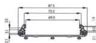
sezione supporto profilato E72-M2 (E72CM) profile support section E72-M2 (E72CM)
